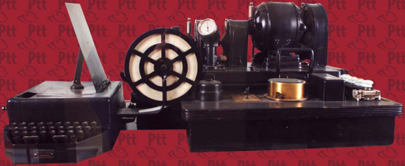
Siemens marka, 110 voltta çalışan, 232 seri nolu, 1912 yapımı elektromekanik hızlı telgraf vericisi (PTT Müzesi)
